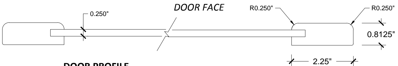
DOOR PROFILE
