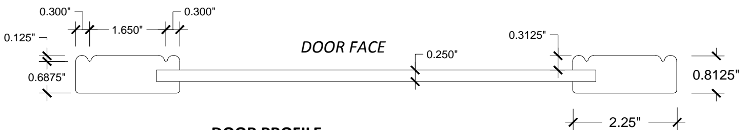
DOOR PROFILE
