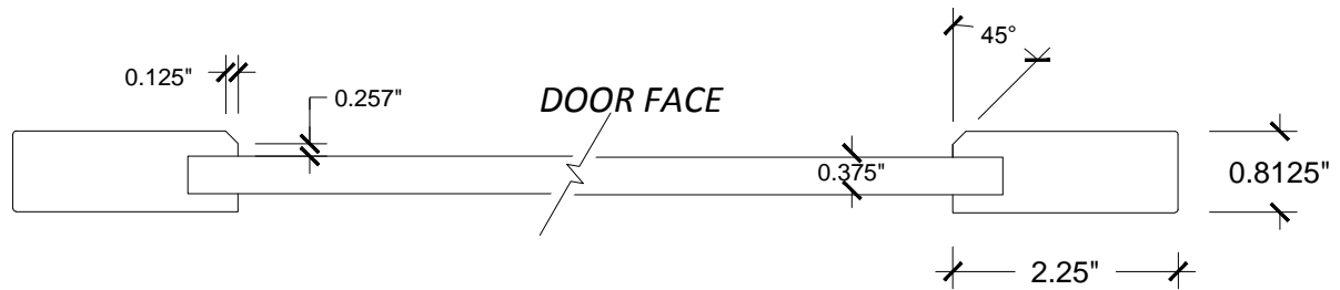
DOOR PROFILE
